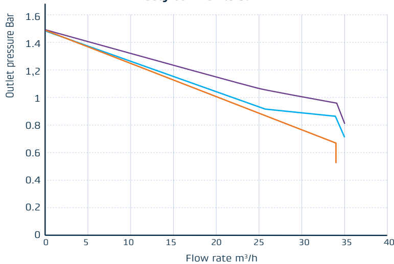
Asetyleeni 25/1.5 bar
